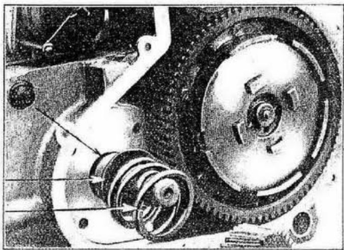
Fig. 40 - Come, tolto il pignone motore, si sfilano le molle di spinta, le ranelle di appoggio e la ranella premistoppa.
