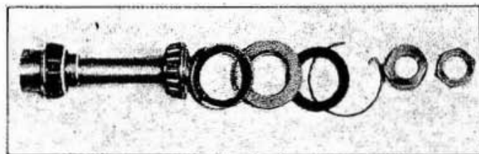
Fig. 87 - Mozzo anteriore. Ordine di montaggio dei vari pezzi.
