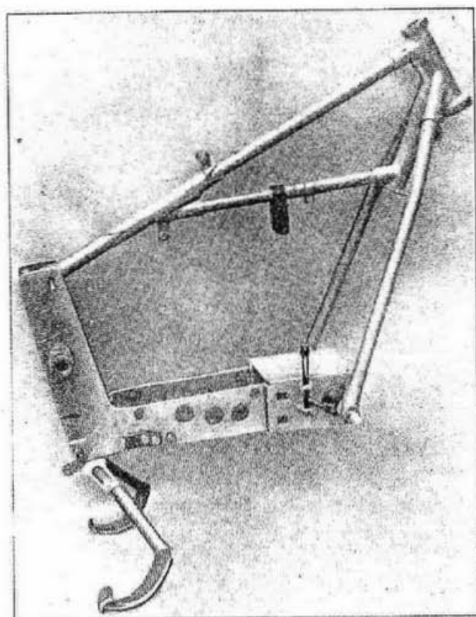
Fig. 31 - Vista del telaio centrale.
