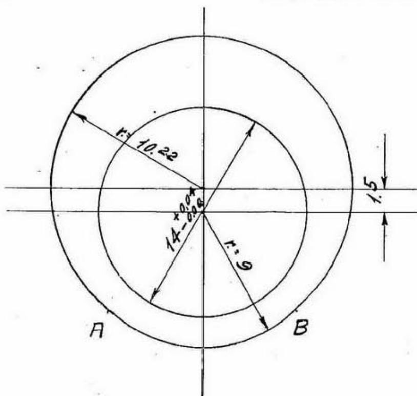
Fig. 73 - Schema sede delle palette.
