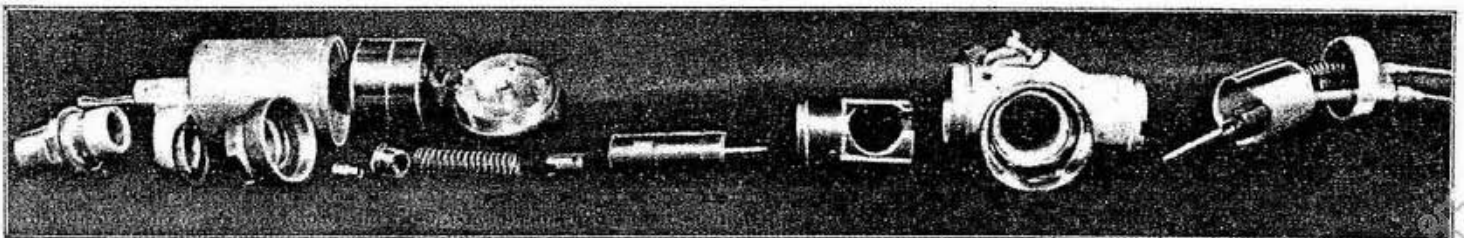
Fig. 67 - Il carburatore smontato.
