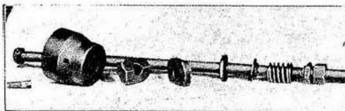
Fig. 86 - Da sinistra a destra: Uno dei 5 bulloncini, la scatola e i blocchetti maschio e femmina. Infilati nel tirante: la ranella di cuoio, il piattello, la molla e il morsetto di fissaggio.
