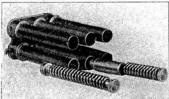
Fig. 84 - Moto biposto. Si notino lo spessore, la molla e la bussoletta di pressione laterali (a sinistra) e centrali.
