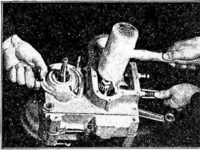
Fig. 46 - Come si apre il carter.
