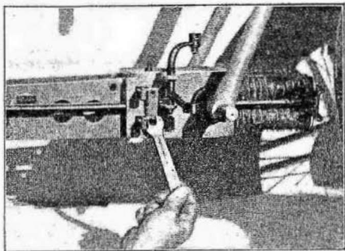
Fig. 25 - Come si leva la pinastitta di fermo delle cremagliere.
