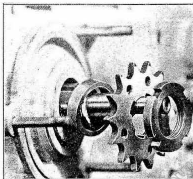
Fig. 45 - Come, dopo allentata la ghiera di serraggio, si levano il pignone e l'anello spessore.
