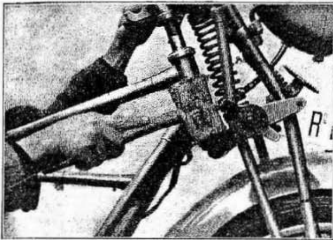
Fig. 29 - Come si sfila il canotto di guida dalla testa di sterzo.
