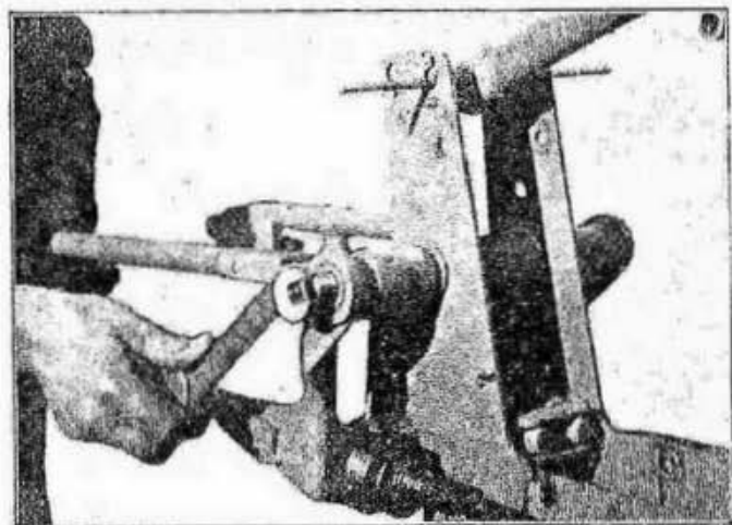
Fig. 26 - Come si leva il perno principale del forcellone oscillante.
