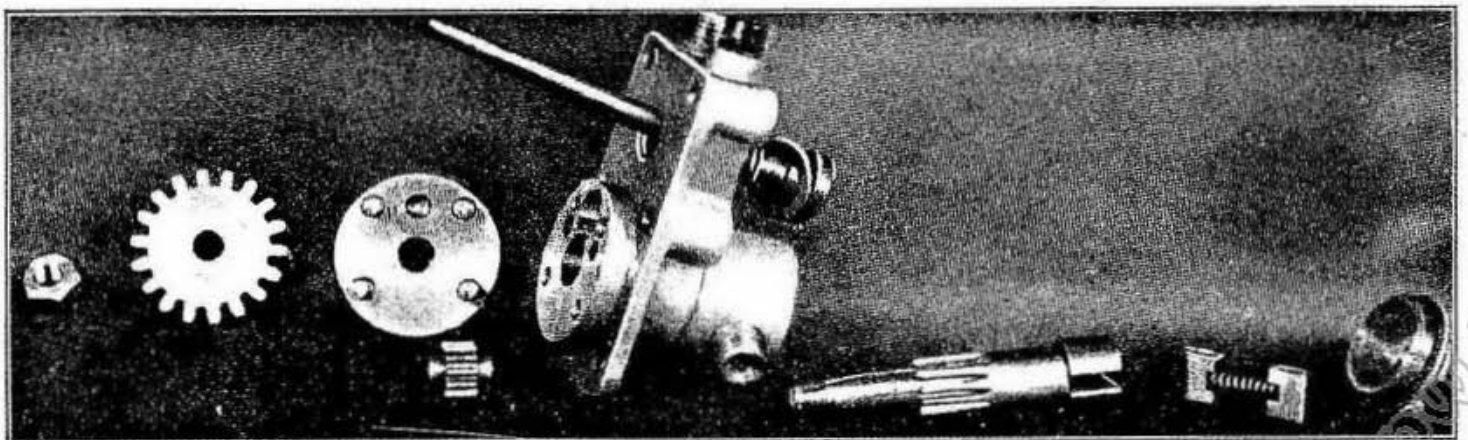
Fig. 70 - La pompa dell'olio smontata. Ordine di montaggio dei singoli pezzi.
