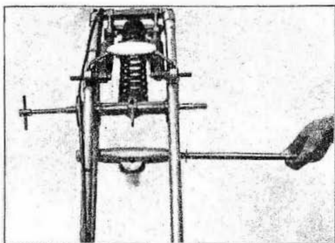
Fig. 35 - Come si levano i perni inferiori. Avvitare completamente e sfilare a sinistra.
