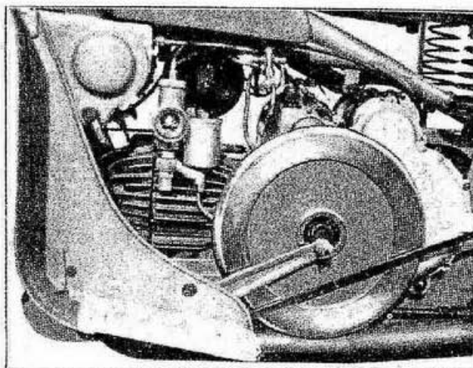
Fig. 4 - Motore montato sul telaio, lato volano.
