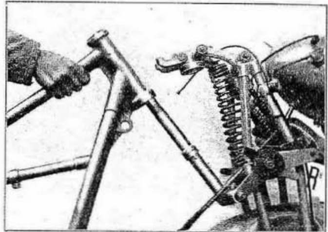
Fig. 30 - Come si sfila il canotto di guida dal canotto del telaio (pipa di sterzo).
