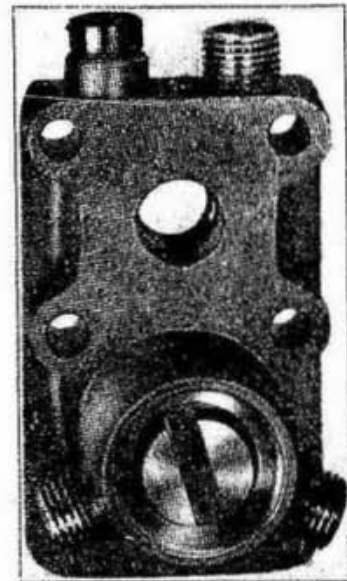
Fig. 72 - Il corpo pompa visto dall'esterno. È visibile la pompa di recupero a palette scorrevoli.
