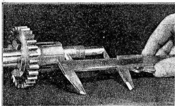
Fig. 63 - Come si misura la distanza fra l'estremità destra dell'albero primario e l'estremità destra dell'ingranaggio presa diretta.
