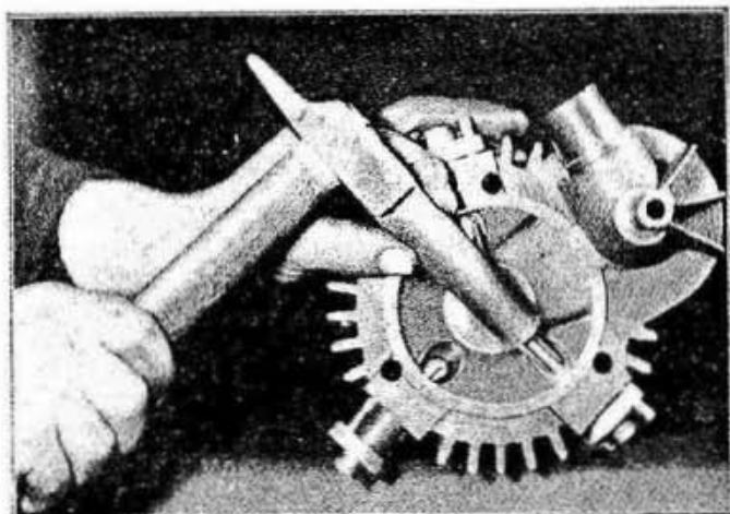
Fig. 52 - Come si levano i paravalvola, quello al basso a sinistra è già stato rimosso.
