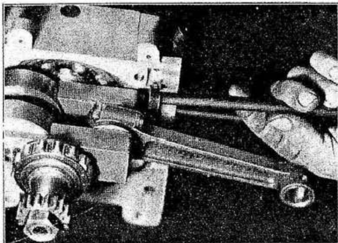
Fig. 75 - Prima di chiudere i due mezzi carter ricordare di piazzare il tirante per fissaggio testa e cilindro.
