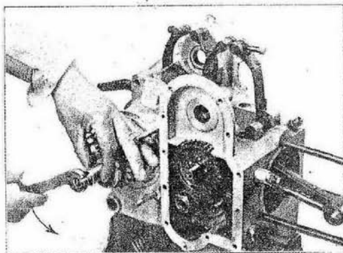
Fig. 42 - Come si leva l'asta interna di comando frizione.
