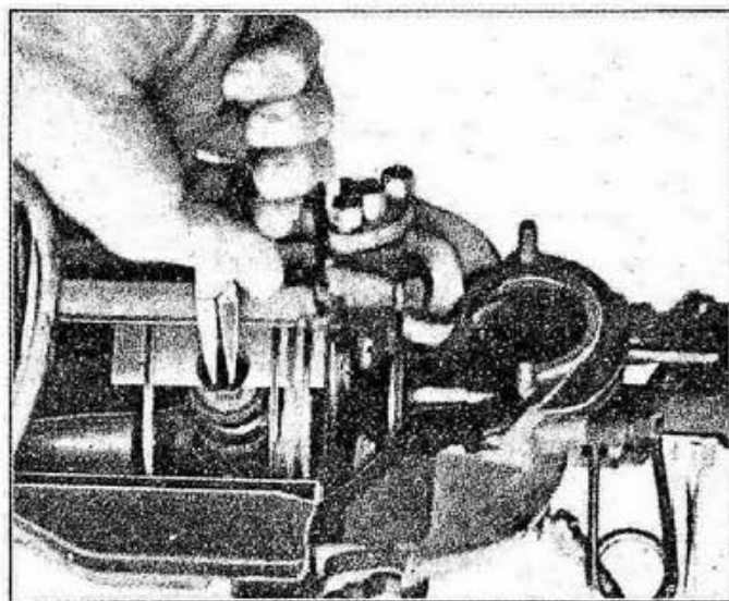
Fig. 39 - Come si leva la molletta (sinistra) che fissa lo spinotto. (Il motore è sezionato).
