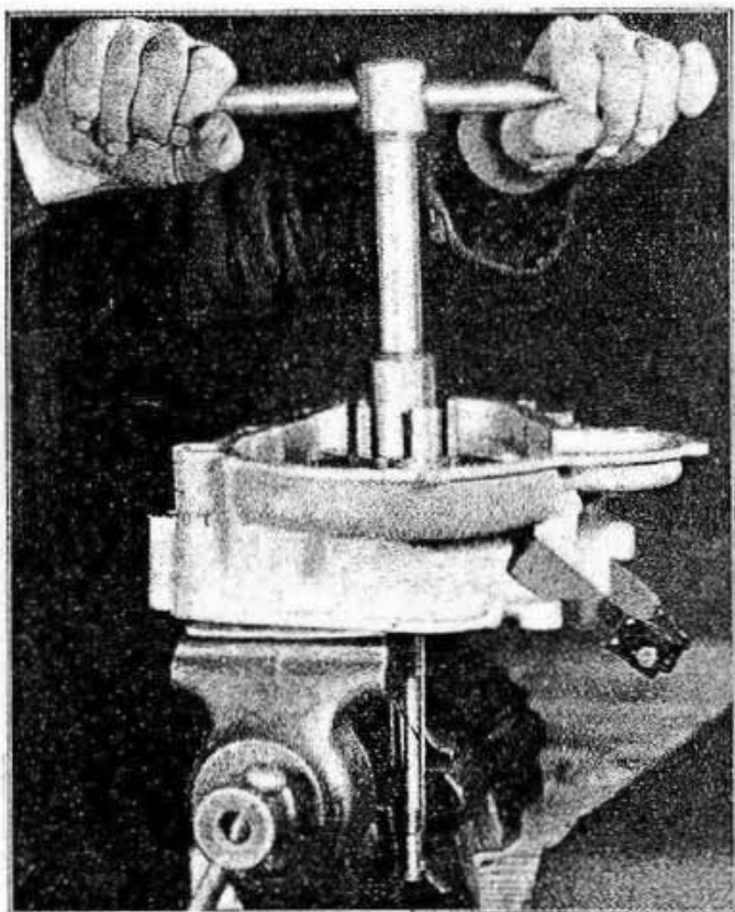
Fig. 50 - Come si prende in mano l'albero primario del cambio e si smontano il controdado e dado di bloccaggio del corpo frizione fisso (griffa).
