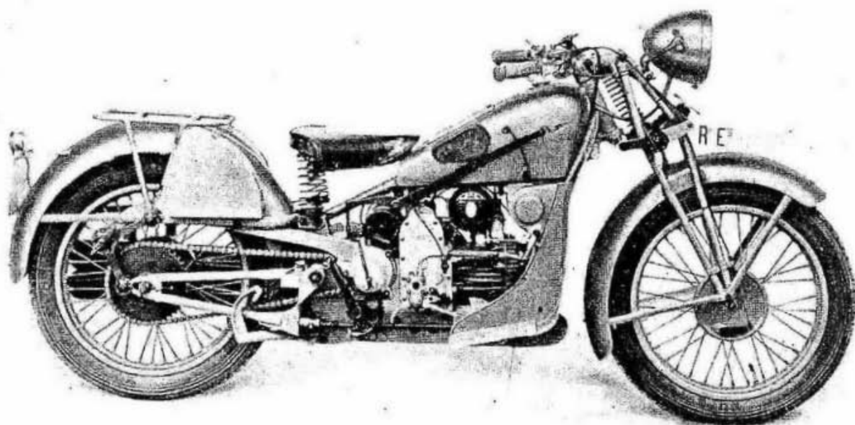
Fig. 8 - Moto "Monoposto" lato distribuzione.
