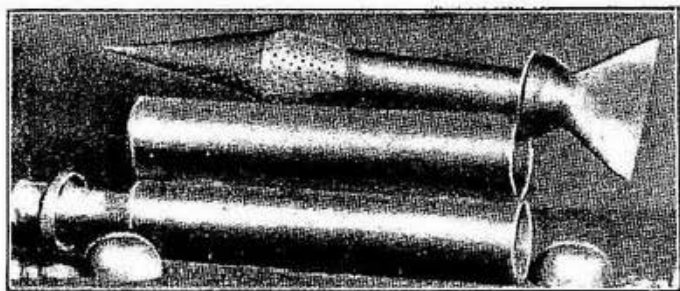
Fig. 68 - Come è formato il silenziatore nelle moto mono e biposto.
