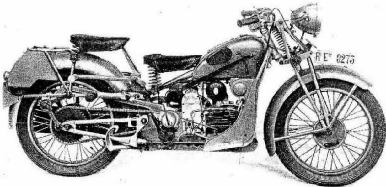
Fig. 12 - Moto "Biposto", lato distribuzione.
