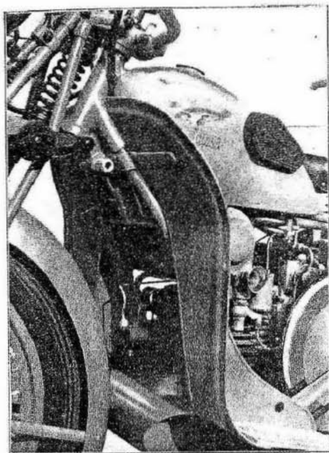
Fig. 9 - Gruppo sterzo - Pedane Scatola coprimolle.
