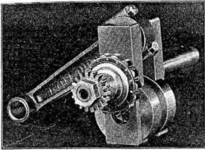
Fig. 56 - Gruppo albero a gomito biella visto dal lato distribuzione. Si notino il dado amussato all'esterno e la bulinatura di sicurezza.
