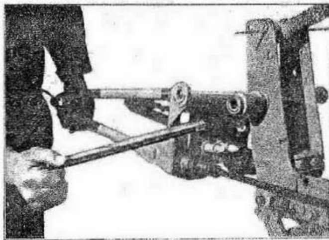
Fig. 28 - Come si leva il forcellone oscillante completo e i tiranti.
