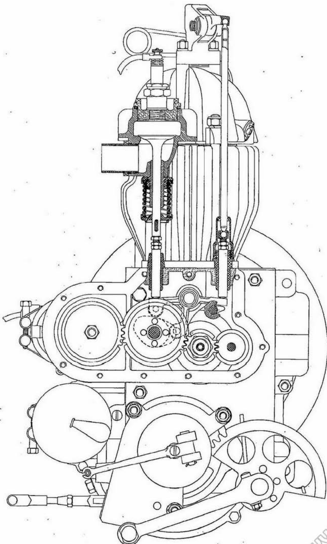
Vista del motore dal lato distribuzione.
