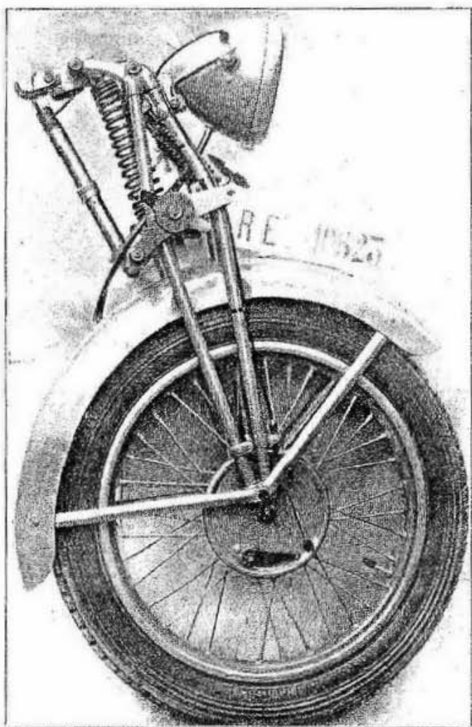
Fig. 33 - Gruppo forcella anteriore completo.
