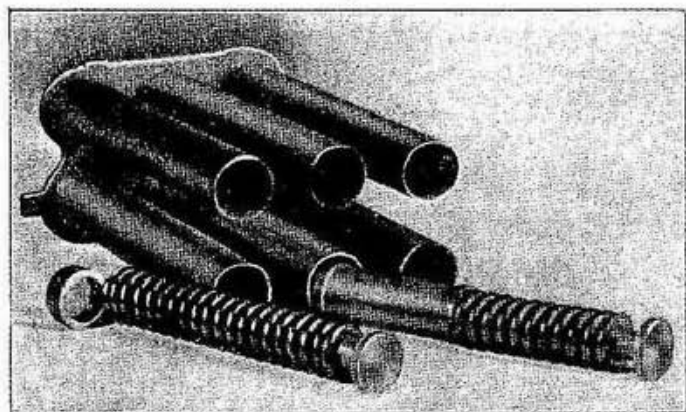
Fig. 83 - Moto monoposto. Si notino la vera spessore, la molla e la bussoletta di pressione laterali (a sinistra) e centrali.
