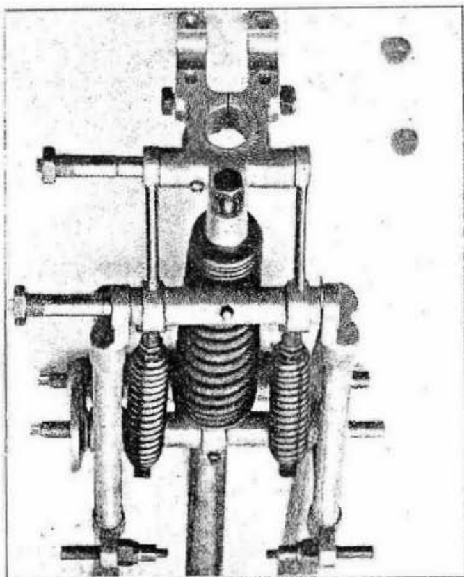
Fig. 36 - Si noti il dado che fissa la molla centrale allentato.
