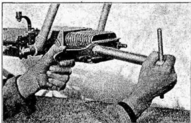
Fig. 21 - Come si leva la piastra premimolle.
