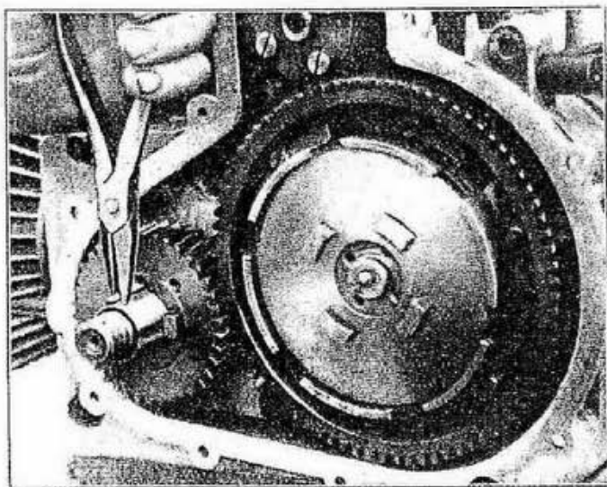
Fig. 41 - Levare la chiave prima di sfilare il pignone motore.
