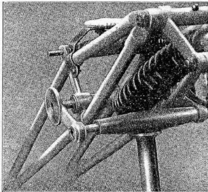
Fig. 37 - Come si leva il biscottino sinistro.
