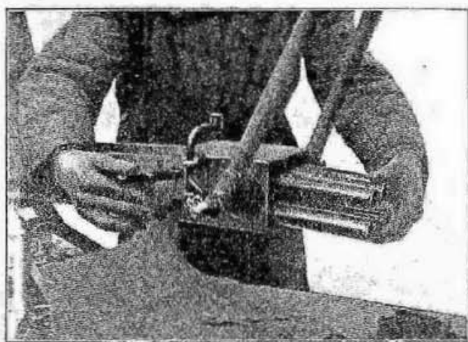
Fig. 27 - Come si levano le due cremagliere e il gruppo tubi reggi molla.
