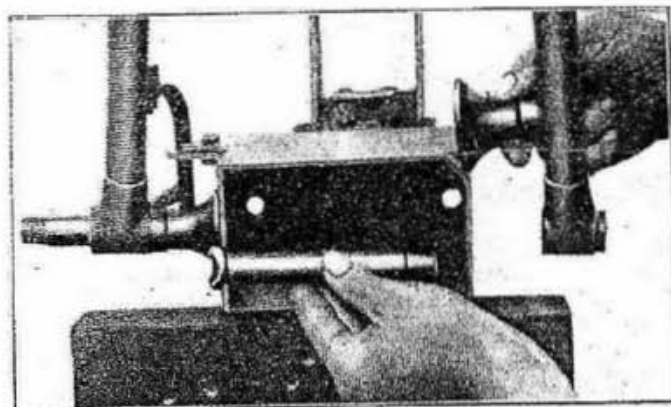
Fig. 32 - Come si levano i due mezzi perni e i rocchetti spessore.
