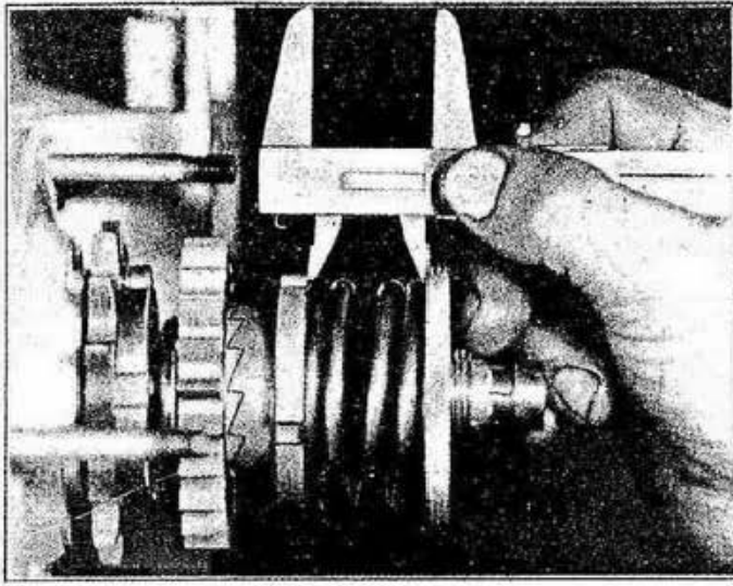
Fig. 62 - Come si regola la tensione delle molle della frizione. La misura normale, come indicato in figura, è mm. 28.
