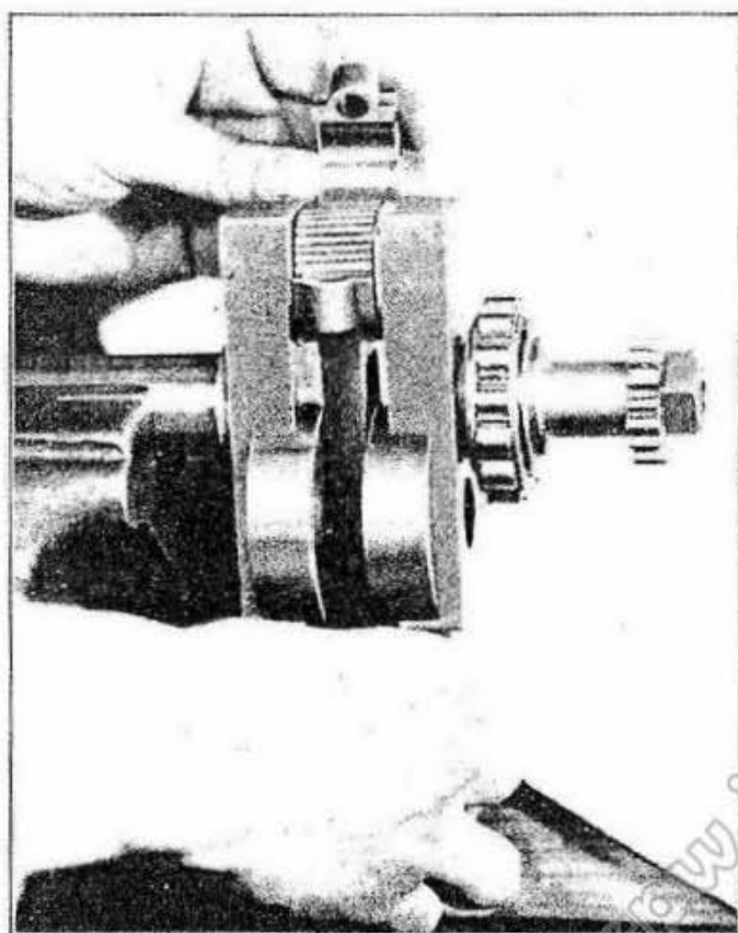
Fig. 59 - Come si montano i rullini della biella.
