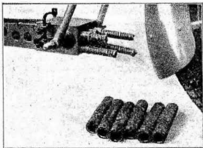
Fig. 22 - Le 6 molle esterne sono già tolte. Si vedono le molle interne parzialmente sfilate.
