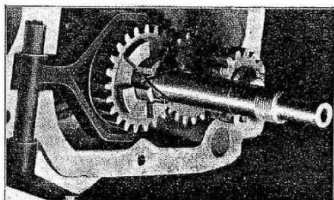
Fig. 64 - La figura mostra l'ingranaggio scorrevole montato sul primario del cambio e forcella con forcellino di ricambio.
