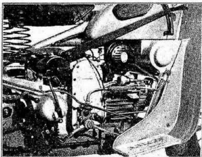
Fig. 3 - Motore montato sul telaio, lato distribuzione.
