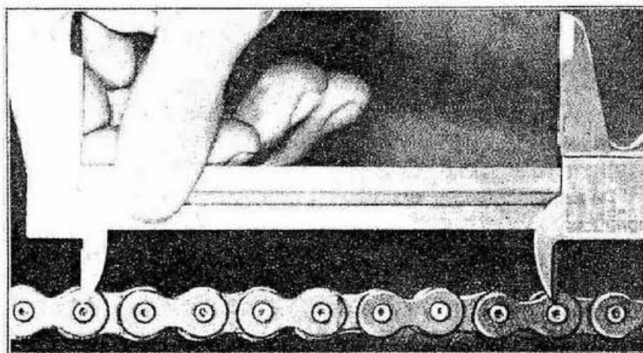
Fig. 66 - Come si controlla l'allungamento della catena di trasmissione.
