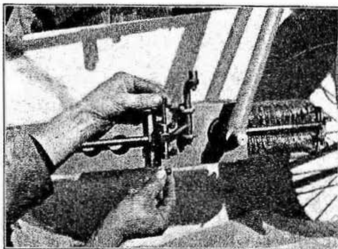
Fig. 24 - Come si leva la vite di tenuta (verticale) delle cremagliere.
