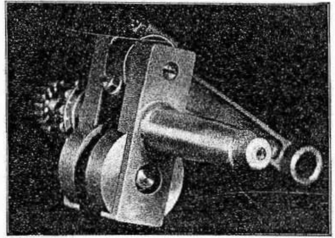
Fig. 57 - Albero a gomito biella visto dal lato volante. Si noti il tappo di ispezione per canale interno dell'olio.
