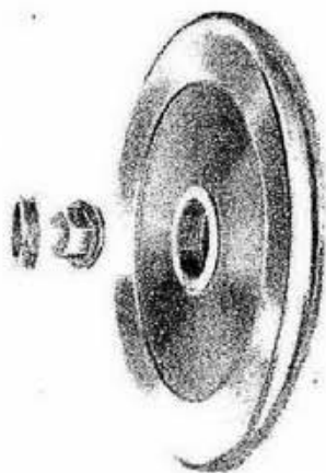
Fig. 13 - Controdado a filetto sinistro. Dado a filetto destro.
