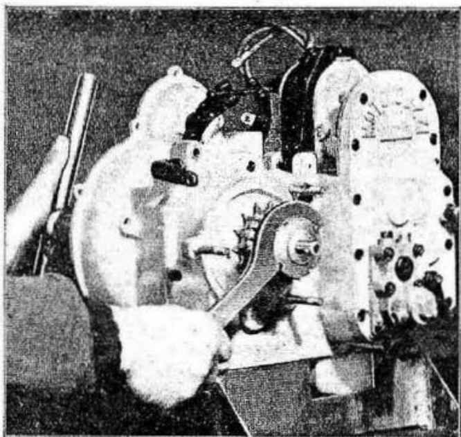
Fig. 43 - Come si smonta il manicotto dentato per la messa in moto.
