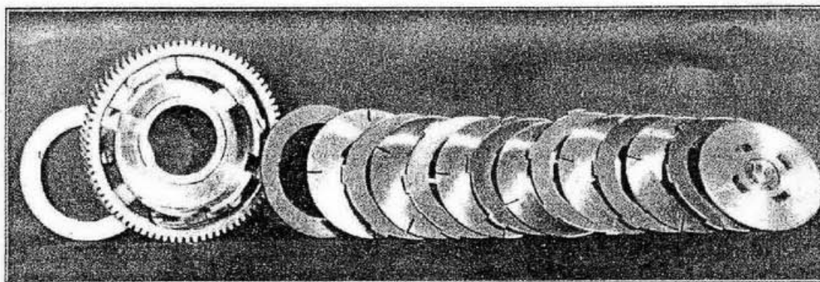
Fig. 61 - (da sinistra a destra - dall'interno all'esterno). Ordine di montaggio dei vari pezzi costituenti la frizione.
