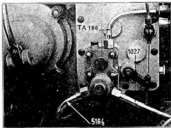
Fig. 15 - Vista della pompa olio e dei tre raccordi: Superiore - Anteriore - Posteriore.
