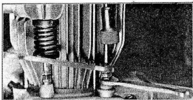
Fig. 77 - Come si regolano le punterie.
