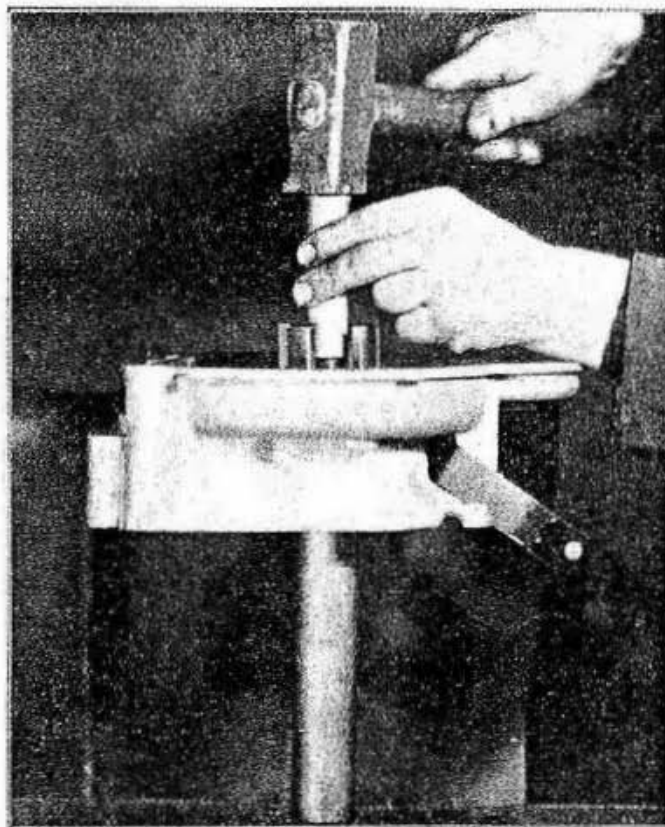
Fig. 51 - Dopo avere infilato sull'albero primario un tubo di ferro, ecco come si sfilava l'albero medesimo.
