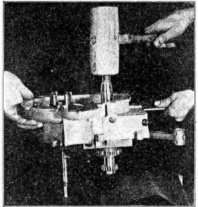
Fig. 48 - Come si leva il gruppo albero a gomito biella. Tenendo sospeso il mezzo carter e battendo dall'esterno verso l'interno.
