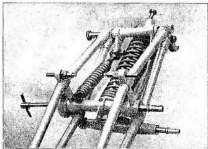
Fig. 34 - Come si levano i perni inferiori.
