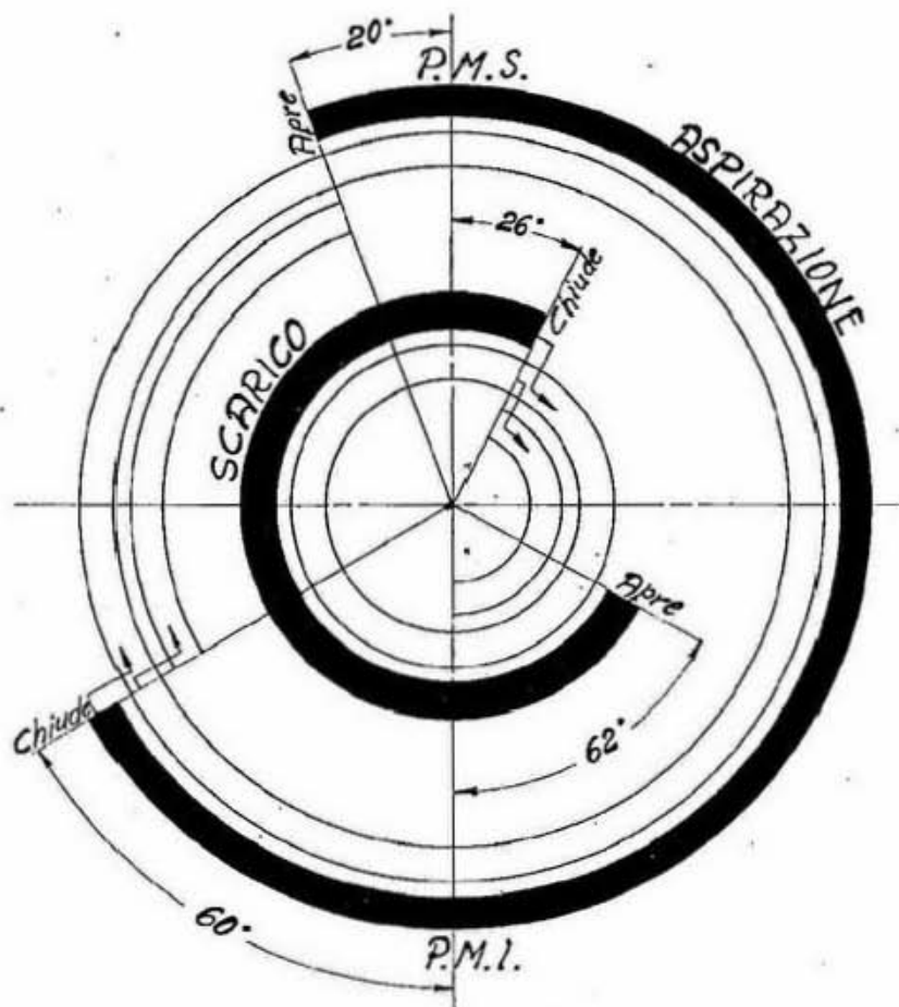
Diagramma angolare di distribuzione riferito all'asse motore
