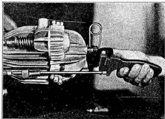
Fig. 76 - Come si monta l'asta di comando per bilancere di scarico.
