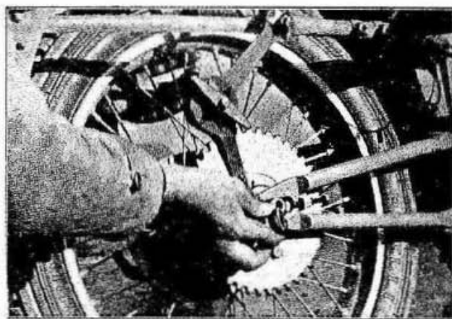
Fig. 20 - Come si leva la ruota posteriore - Il perno è già stato sfilato - Si vede nella mano il dado per perno forato.
