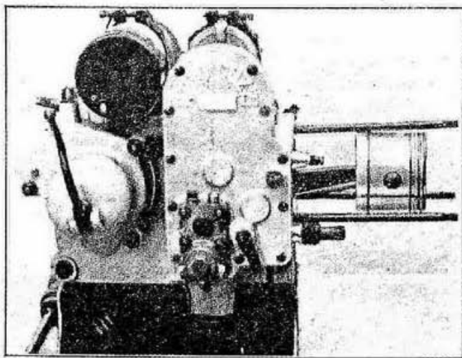
Fig. 38 - Motore senza cilindro e testa.
