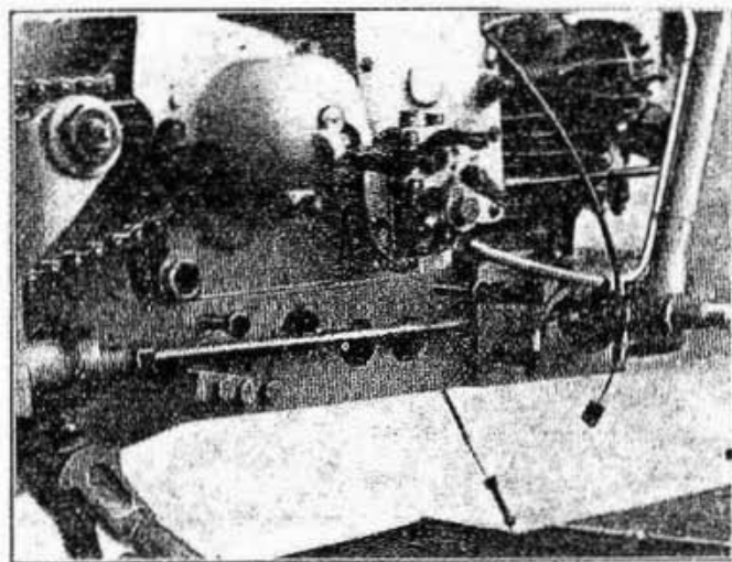
Fig. 16 - Sono visibili i due bulloni che fissano inferiormente il carter alle piastre porta motore.
