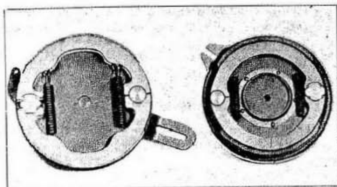
Fig. 89 - Piatto portaceppi posteriore e anteriore.
