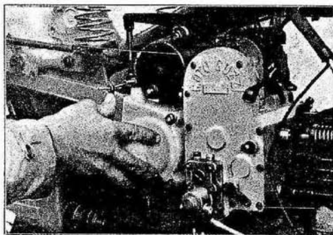
Fig. 14 - Come si smonta il comando della frizione.
