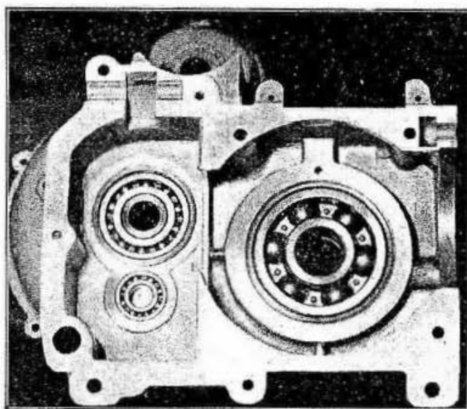
Fig. 49 - Vista interna del mezzo carter sinistro (lato volano). Si notino il cuscinetto a sfere (grande) per albero motore, il cuscinetto piccolo per albero secondario cambio e il cuscinetto per albero primario. Si noti che in quest'ultimo è ancora montato il corpo frizione liscio (anello interno) che si estrae battendo dall'interno verso l'esterno sull'albero cavo (conico).
