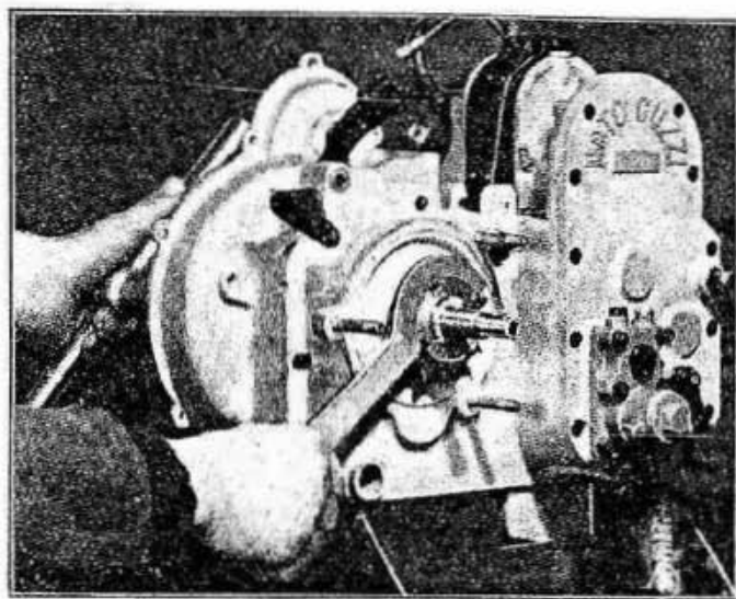
Fig. 44 - Come si smonta la ghiera di serraggio del pignone del cambio.
