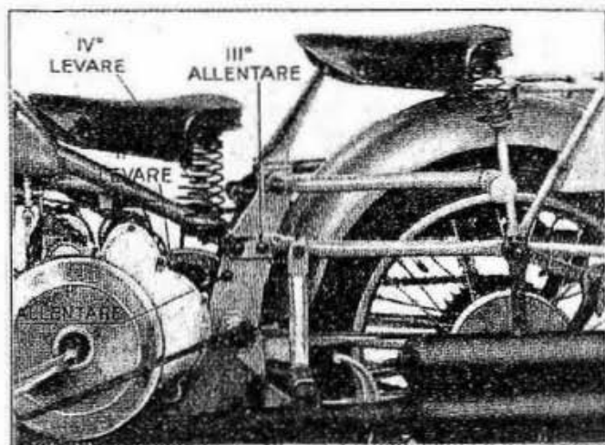
Fig. 17 - Le ultime operazioni da eseguirsi per aprire il telaio e togliere il motore.
