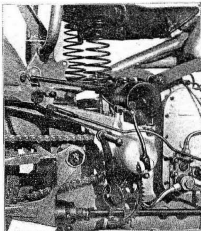
Fig. 10 - Moto biposto - Gruppo frizione - Avviamento Pompa olio. Sono visibili in basso i tiranti del forcellone oscillante.
