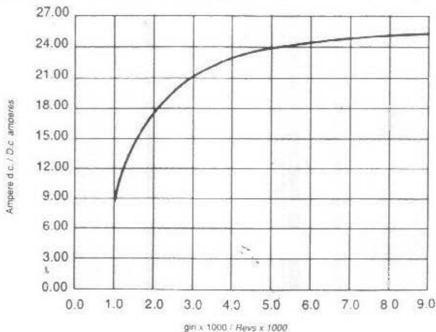
Grafico intensità corrente di carica (2ª serie)
